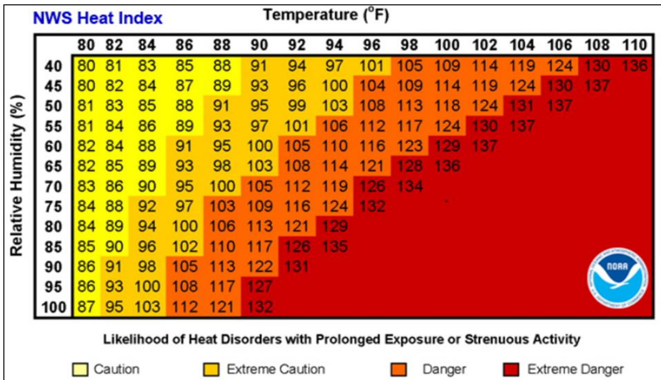
Figura 10-2. Gráfico del índice de calor del NWS: áreas sombreadas
