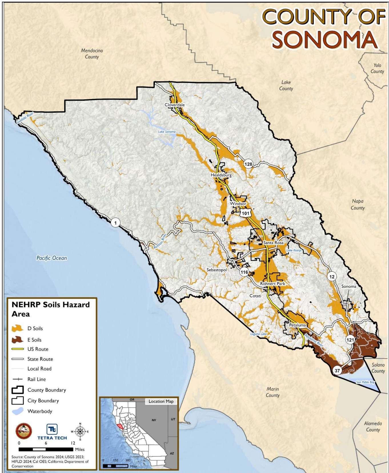
Figura 8-1. Áreas de suelos de clase D y E según NEHRP en el Condado de Sonoma
