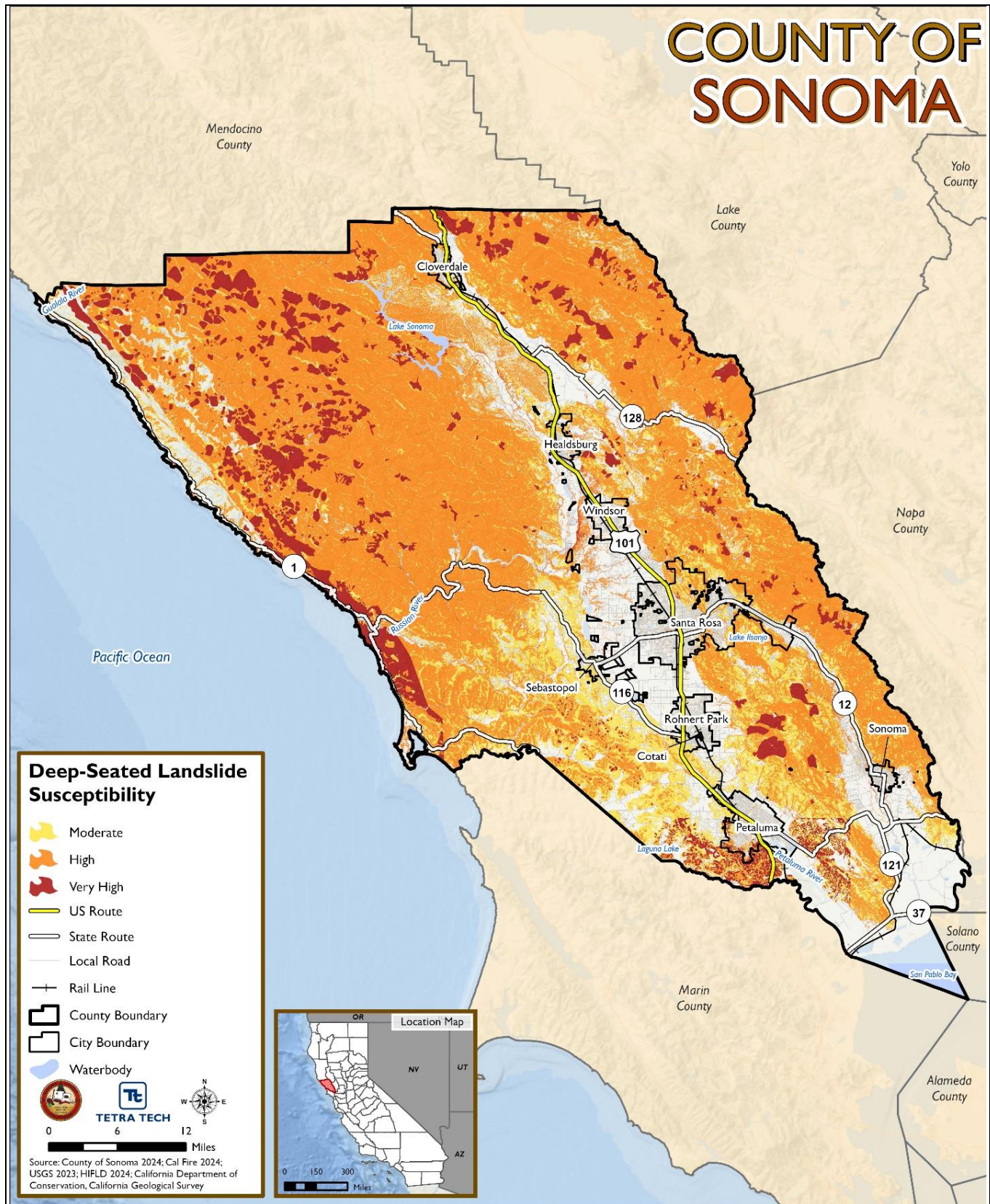
Figura 13-1. Susceptibilidad a deslizamientos de tierra profundos
