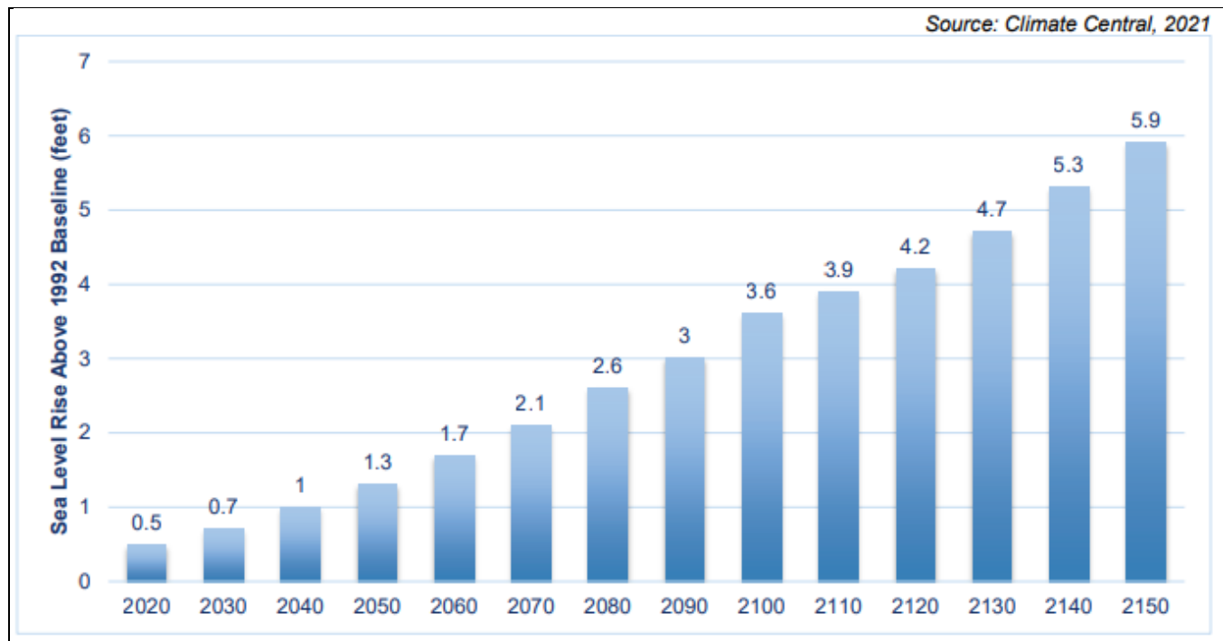
Figura 14-2. Proyección intermedia del aumento del nivel del mar en el condado de Sonoma por encima de la línea base de 1992
