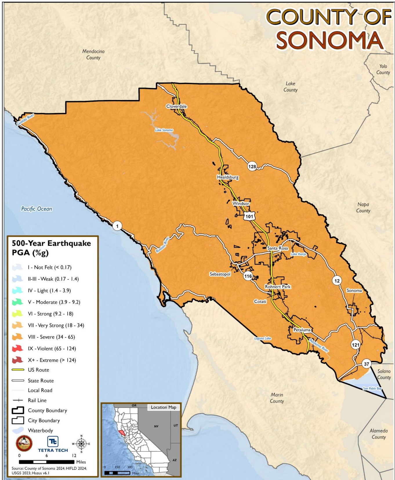
Figura 8-2. Impactos de un terremoto con período de retorno de 500 años en el Condado de Sonoma
